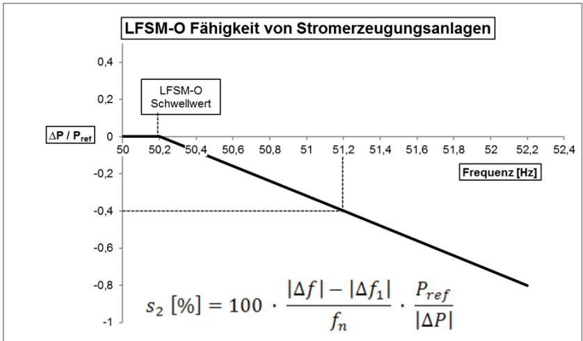
Abbildung 1: Fähigkeit von Stromezeugungsanlagen zur frequenzabhängigen Anpassung der Wirkleistung im LFSM-O-Modus
