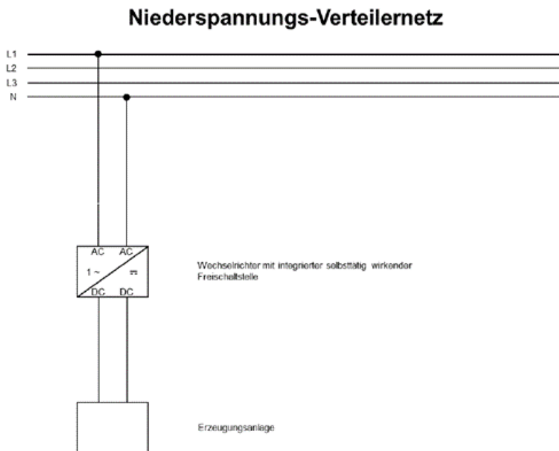
Abbildung 18: Netzanschluss bei Einsatz einer selbsttätig wirkender Freischaltstellen für einphasige Wechselrichter (max. 3,68 kVA)
