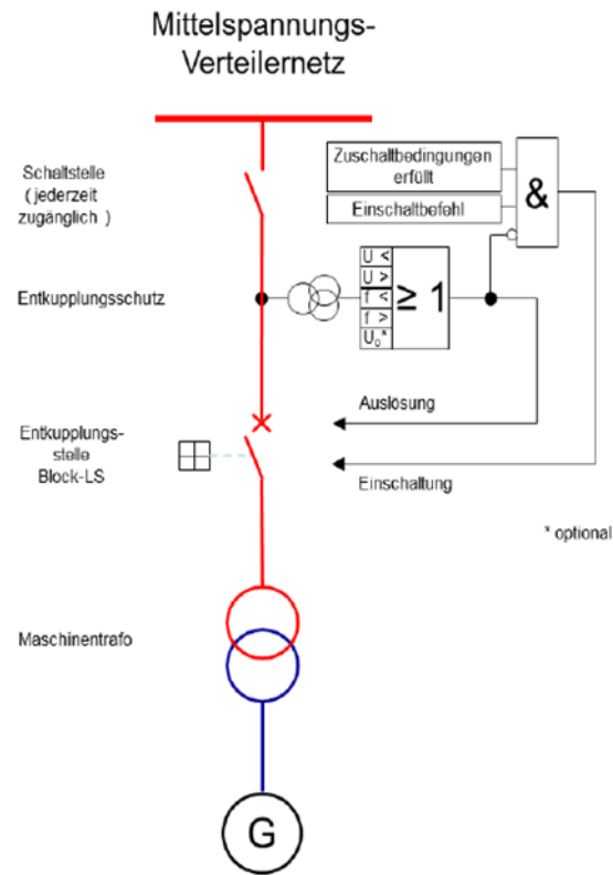
Abbildung 17: Netzanschluss an das Mittelspannungsnetz mit Netzentkupplungsschutz
